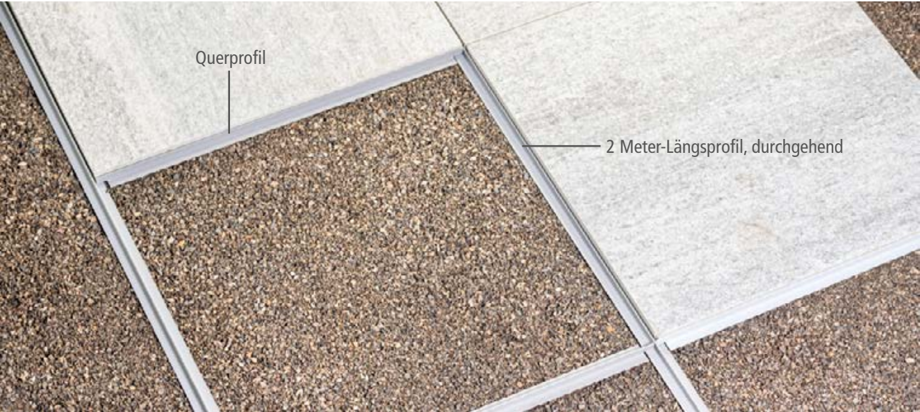
Die Querprofile lassen sich nachträglich unter die Platte schieben.
