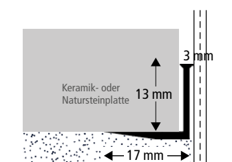
L-Profil für Fassadenanschluss
