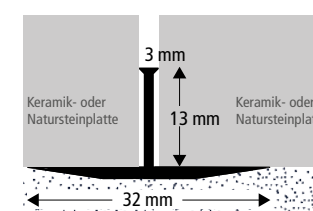
Fugenprofil
