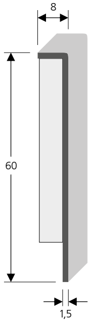
Typ B 056
