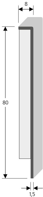
Typ B 056
