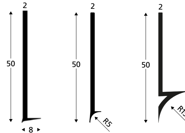
Mit R5-Profil
